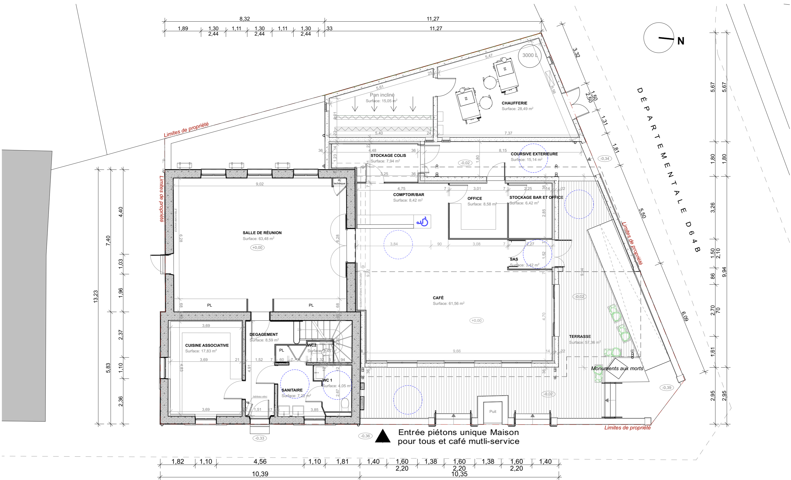
Plan Rez-de-chaussée - Projet - Ech 1/100e
